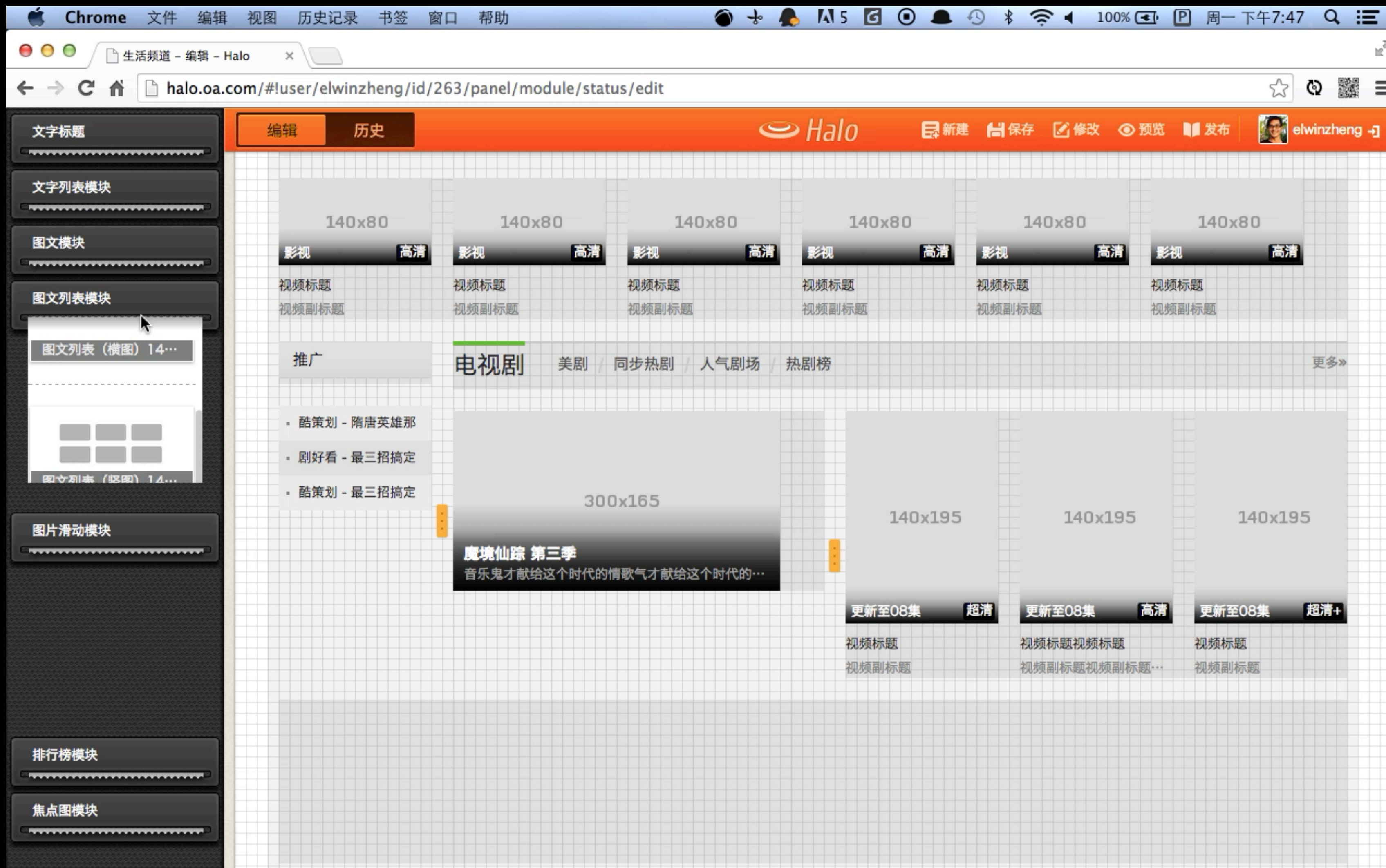
组件拖拽的页面生成工具
